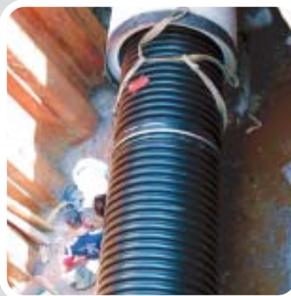
PKS-Kanalrohr DN 1400 - Rohrstranganierung
