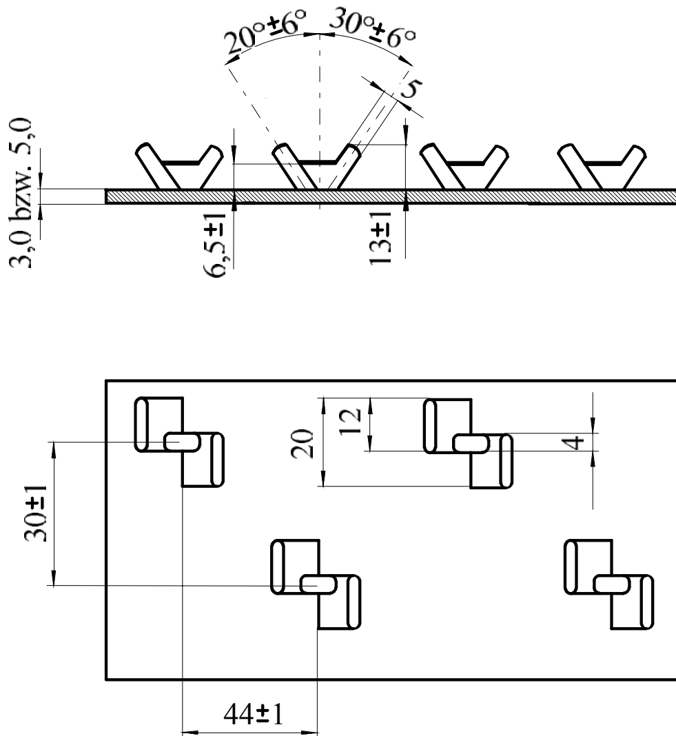
Figur 3: Inliner mit homogen, aus Grundmaterial ausgeformten Ankernoppen
