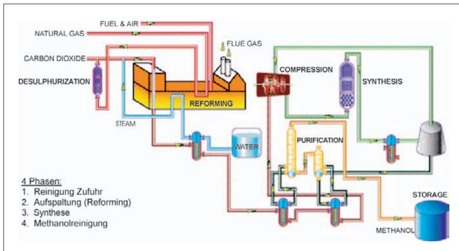
Bild 1: Produktion von Methanol
